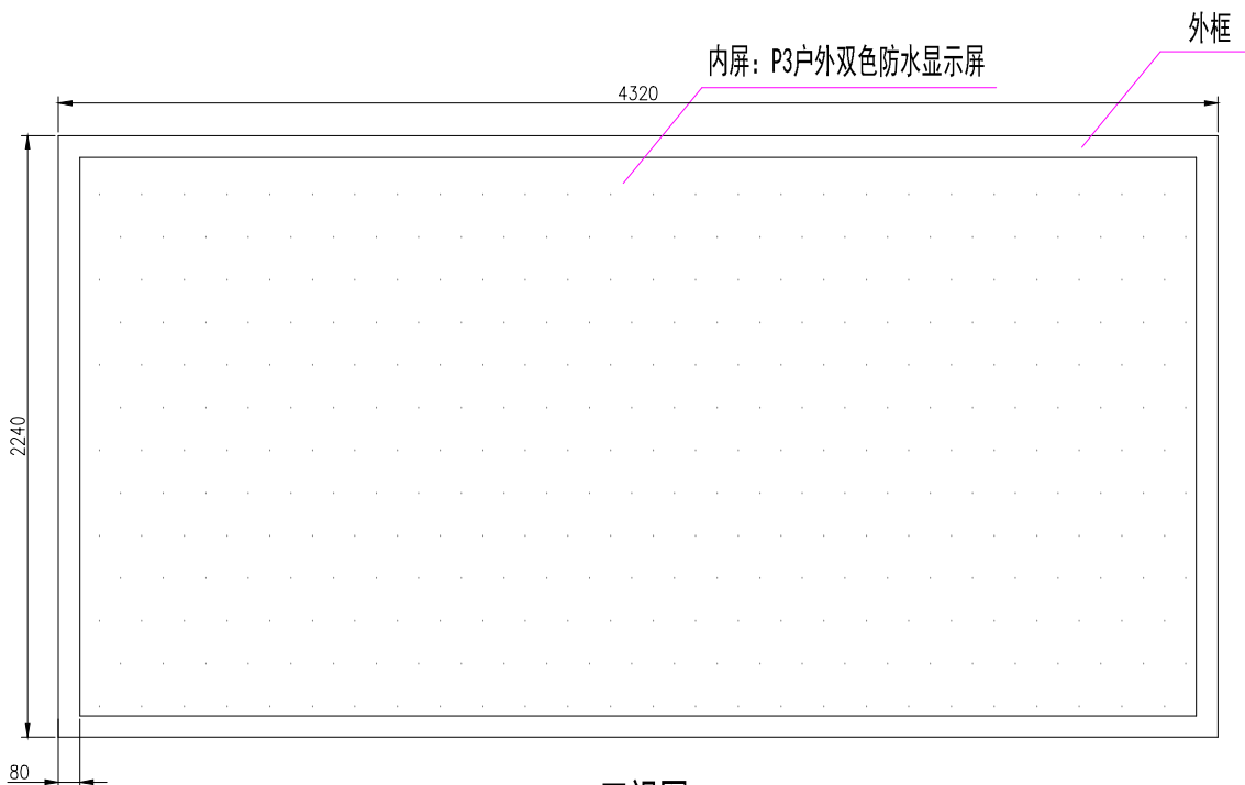
正视图
