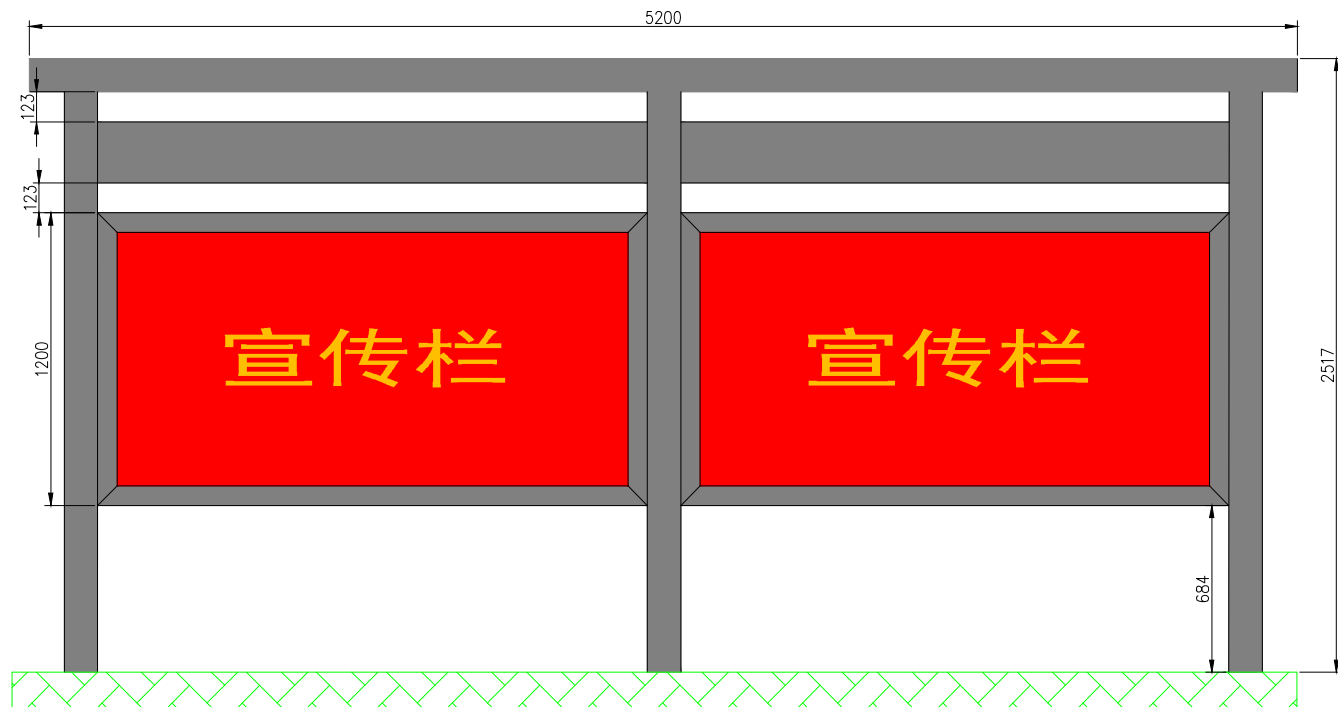
正视图
